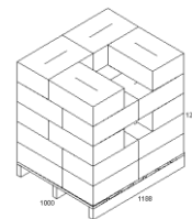
Paletógrafo Recomendado
